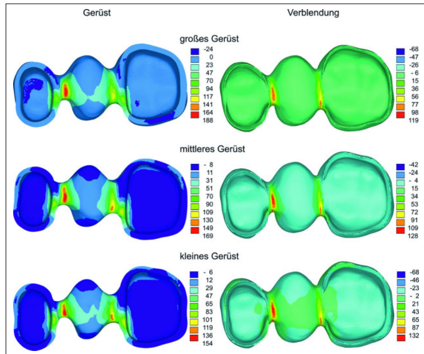
Abbildung 4 Erste Hauptnormalspannung (MPa) im Gerüstwerkstoff (links) und in der Verblendkeramik (rechts) für den Lastfall 2 bei von oben nach unten abnehmender Gerüstgröße.
