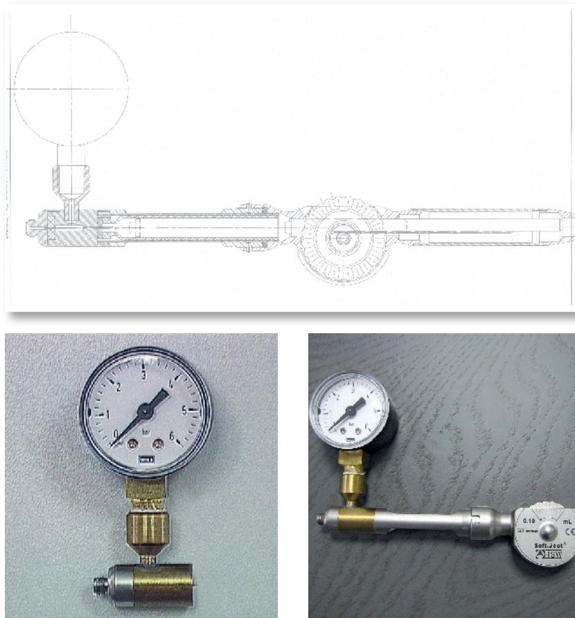
Abbildung 2a-c SoftJect-Dosieradspritze in Kombination mit Druckmessgerät mit Rohrfeder der Firma WIKA, Klingenberg, gemäß Zeichnung V-1918-01.
