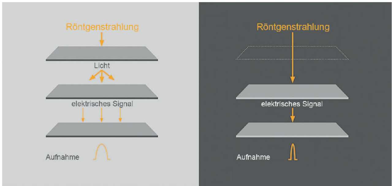
Abbildung 3a Schema eines Sensors mit fluoreszierender Schicht; 3b Schema eines CDTe Sensors ohne fluoreszierende Schicht. Mit diesem wird bei niedriger Dosis eine hohe Zeichenschärfe und bessere Bildqualität erreicht. (Abbildungen umgezeichnet nach Sirona)
